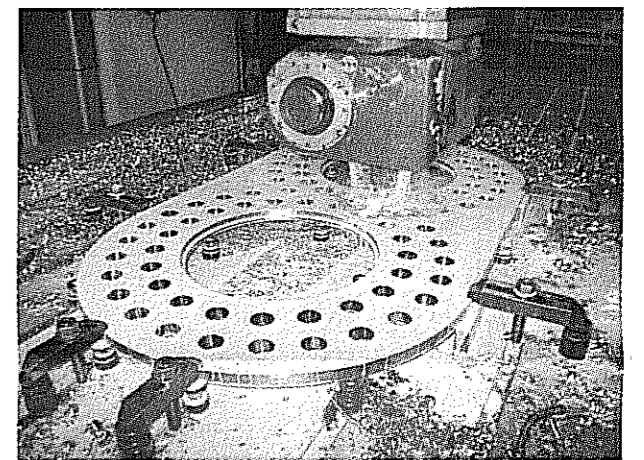
ハルドックス600の穴明け加工
