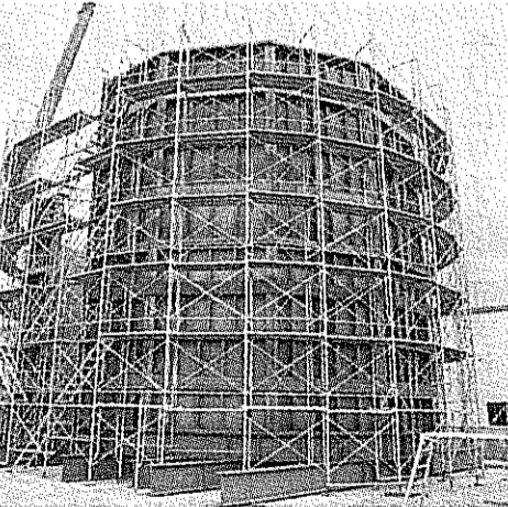
ダム改修に使う仮設構造物の仮組み
